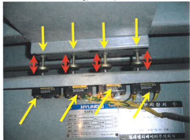
120번[ 과부하장치(오버로드) ]/₩14,500원
