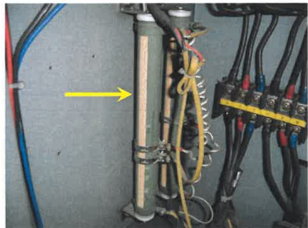
30번 [ 브레이크 막대 저항 ] / ₩80,000원
