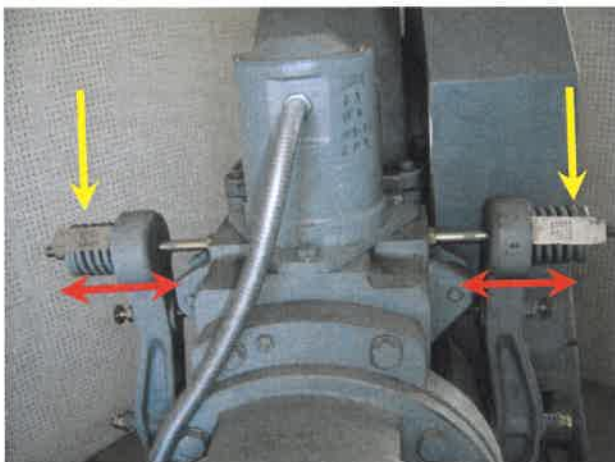
51번[ 브레이크 스프링 ]/₩52,000원
