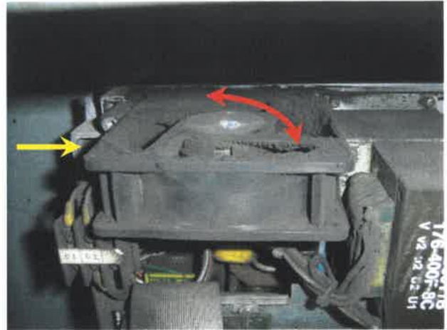
38번[ 인버터 FAN ]/₩53,000원
