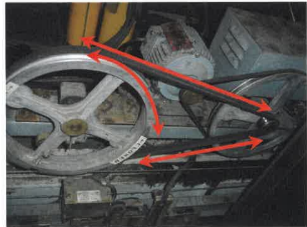
78번[ 카 도어 벨트( 풀리 축 ) ]/₩21,000원
