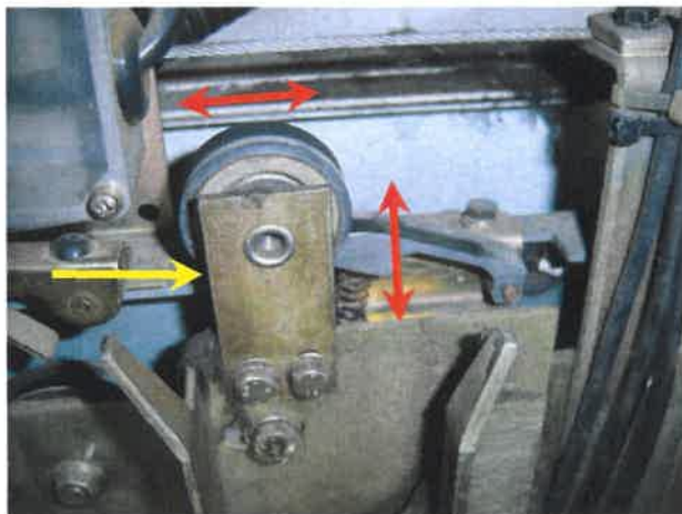
89번[ 카 도어 달침 홀더 ]/₩29,000원
