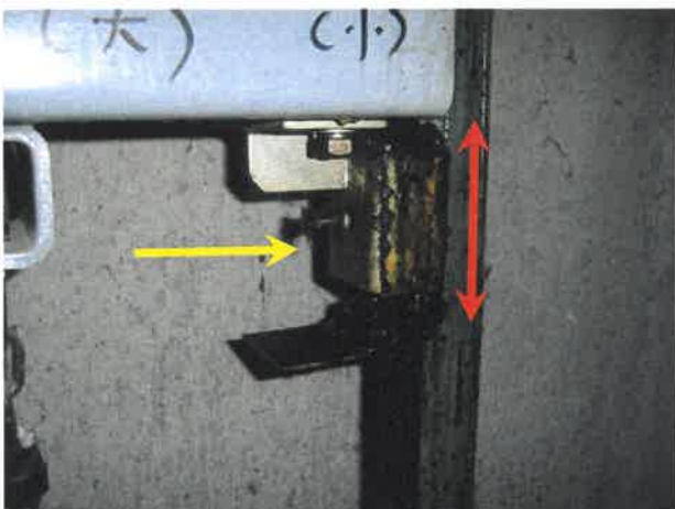
141번[카운터(균형추) 가이드 슈]/₩170,000원
