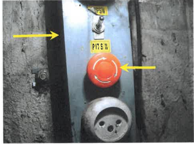
152번[ 피트/E STOP스위치/박스 ]/₩176,000원 [교체주기 : 2년]
