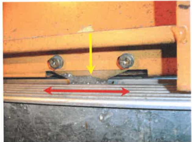
134번[ 도어 가이드 슈 ]/₩6,820원 [교체주기 : 1년]
