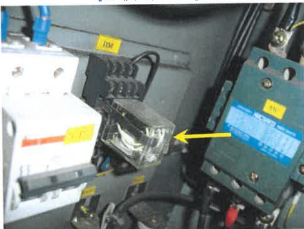
29번[ 마그네트(MC) 보조 릴레이 ]교체주기 : 1년] 오므런 ₩77,000원 / 금성 ₩66,000원
