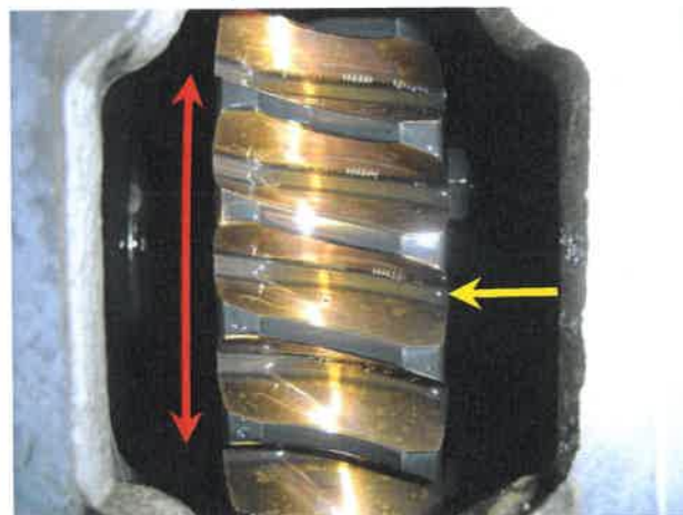
59번[ 웜기어 ]/₩3,850,000원 [교체주기 : 10년]
