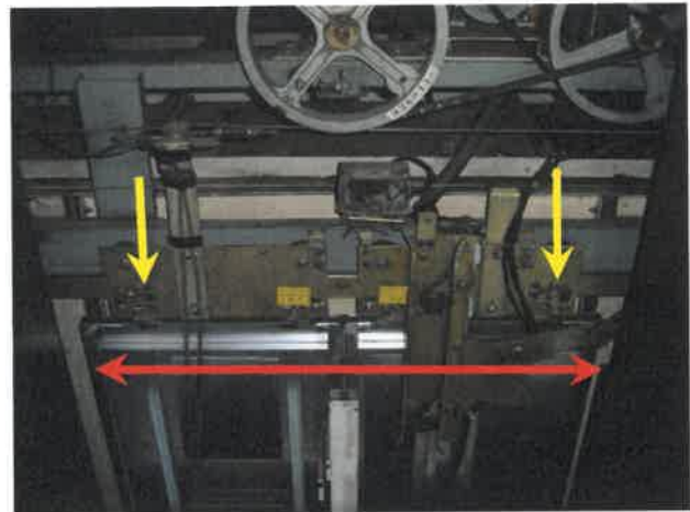
80번[카 도어 행거 플레이트]/₩396,000원/1SET [교체주기 : 3년]
