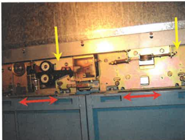
129번[ 도어 행거 플레이트 ]/₩277,200원/SET [교체주기 : 5년]
