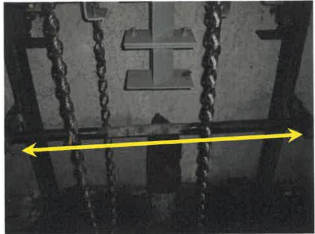
146번 [ 벨런스 체인가이드 슬타입 ] / ₩1,163,800원 [교체주기 : 3년]
