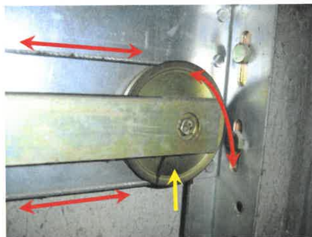
131번[ 도어 연동롤러 ]/₩68,200원 [교체주기 : 5년]
