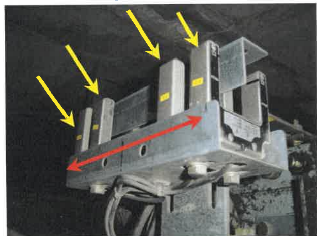
102번[ 착상 장치 ]/₩145,200원 [교체주기 : 3년]
