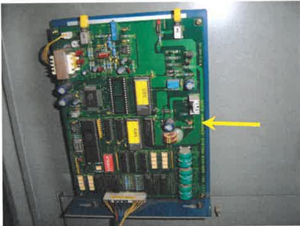
15번 [ 자동음성 안내방송 PCB ] / ₩880,000원 [교체주기 : 5년]
