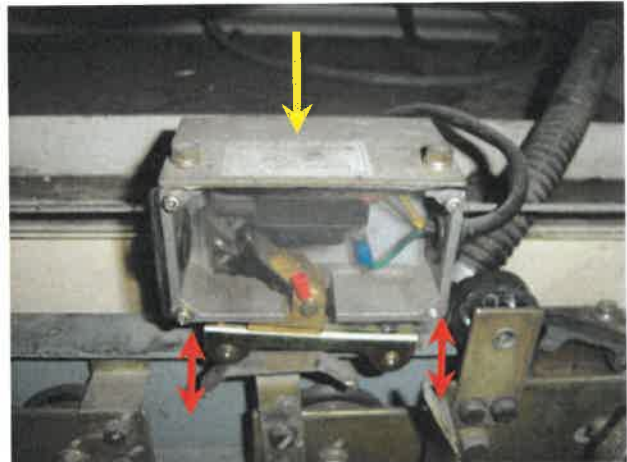
88번[ 카 도어 게이트 스위치 ]/₩154,000원 [교체주기 : 2년]
