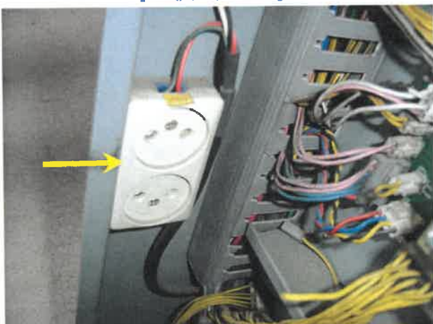
35번[ 제어반 콘센트/AC220V ]/₩13,200원 [교체주기 : 2년]
