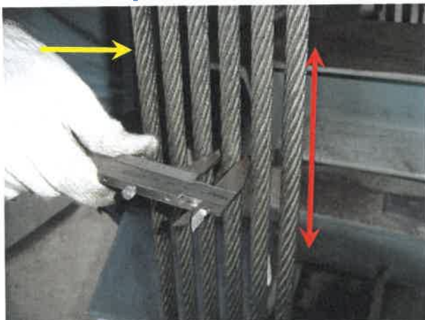
53번[ MAIN 와이어 ROPE ]/1M단위:₩6,198원 [교체주기 : 5년]
