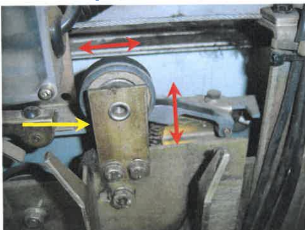
89번[ 카 도어 닫힘 롤러 ]/₩82,500원 [교체주기 : 2년]
