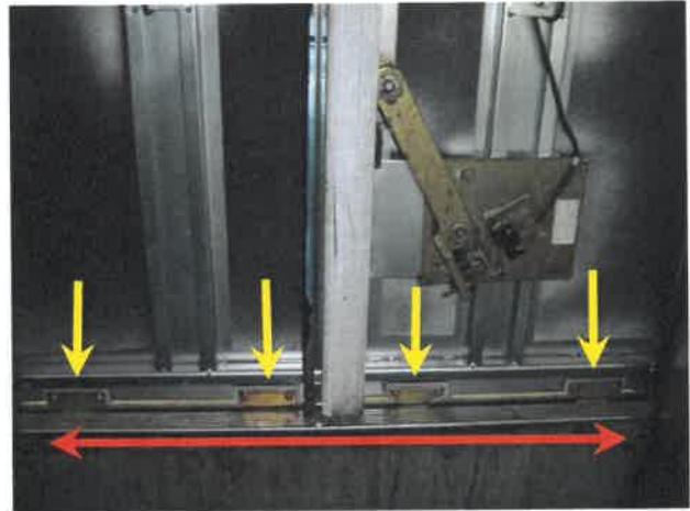
86번[ 카 도어 가이드 슈 ]/₩6,820원 [교체주기 : 1년]
