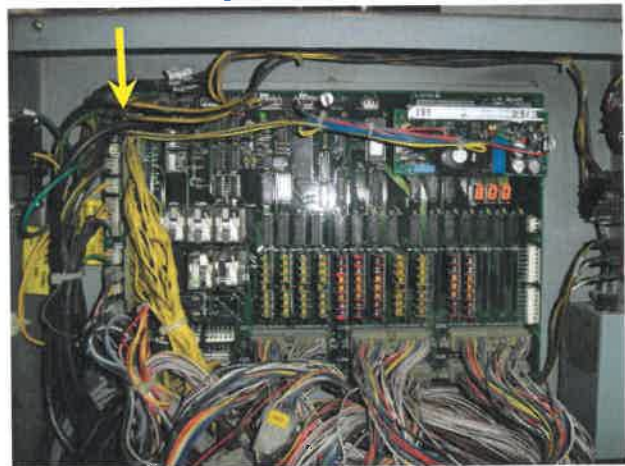
12번[카 상부 통신제어 PCB(CTB)]/₩3,850,000원 [교체주기 : 7년]
