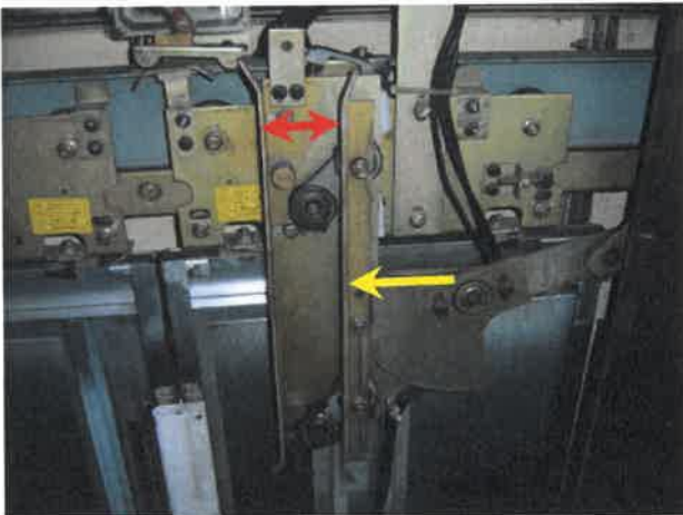
87번[ 카 도어 벤 클러치 ]/₩1,012,000원 [교체주기 : 15년]
