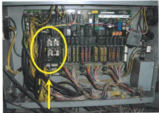
70번[ 카 안전 릴레이 ]/[교체주기 : 1년] 오므런 ₩77,000원 / 금성 ₩66,000원
