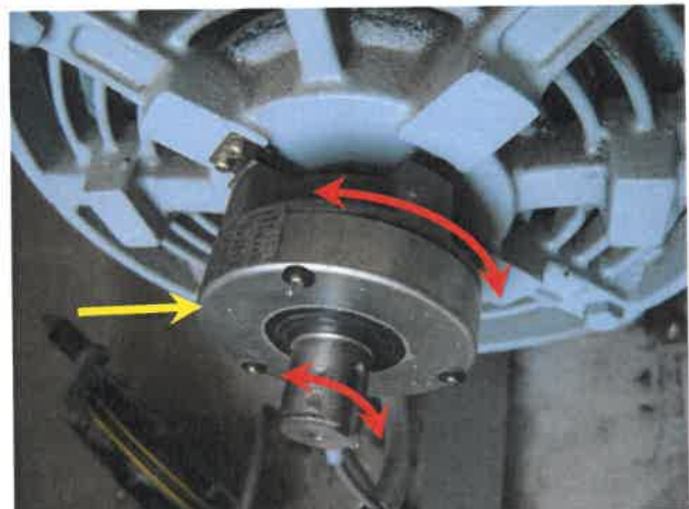
40번[ 속도 검출기(로타리 엔코더) ]/₩900,000원 [교체주기 : 3년]
