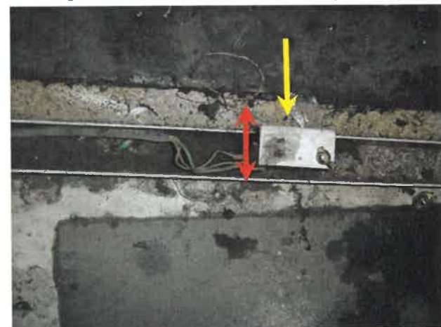
96번[ 카 상부 비상구 스위치 ]/₩35,200원 [교체주기 : 2년]
