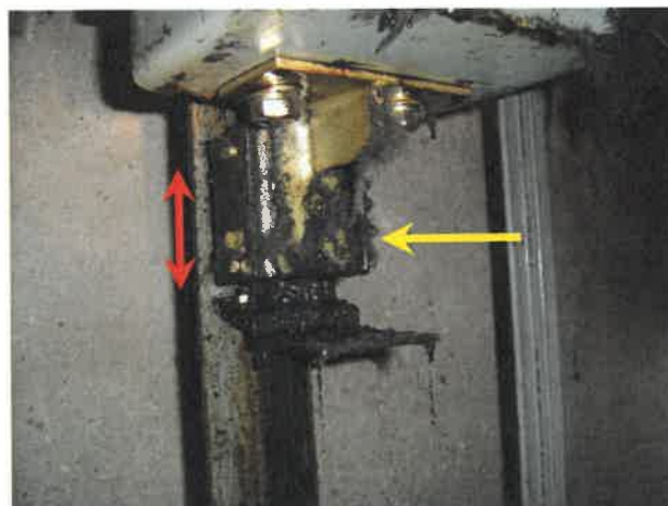
95번[ 카 가이드 슈-상부/하부 ]/₩385,000원롤러 [교체주기 : 5년] 슈타입:₩148,500원
