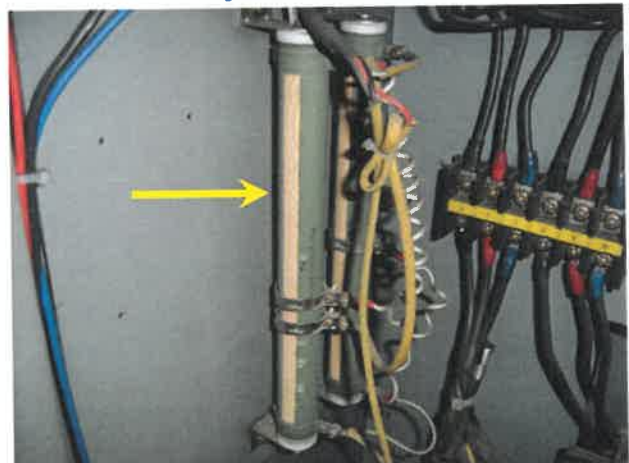
30번[ 브레이크 막대 저항 ]/₩165,000원 [교체주기 : 5년]
