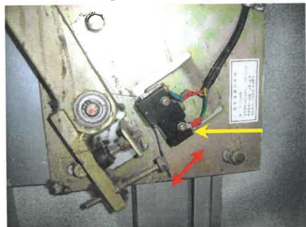
84번[ 세프티 슈 마이크로 스위치 ]/₩35,200원 [교체주기 : 3년]
