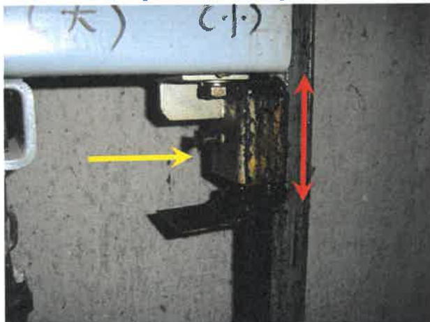
141번 [카운터(균형추) 가이드 슈]/₩275,000원 [교체주기 : 5년]
