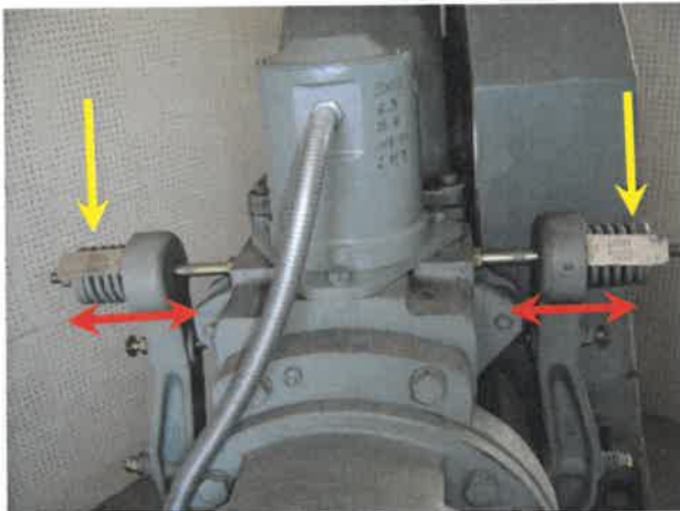
51번[ 브레이크 스프링 ]/₩79,200원 [교체주기 : 10년]
