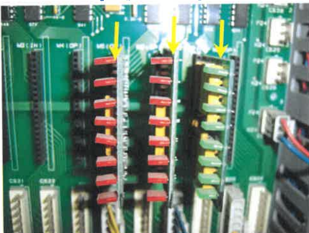
17번 [ 비상용 층 제어 신호 모듈 ] / ₩132,000원 [교체주기 : 5년]
